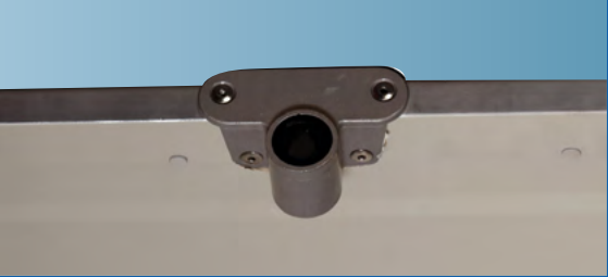
[L-SG1022] Oarlock holder / Rudergabelnhalter
